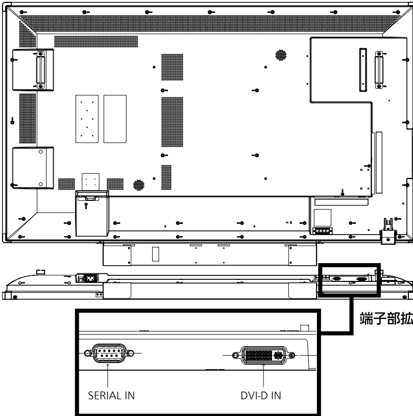
端子部 a 断面図 SERIAL IN/DVI-D IN
